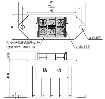
M-2A形 質量：約100g
