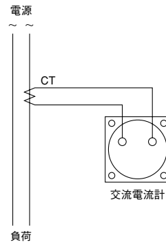
CTと組合せる場合
