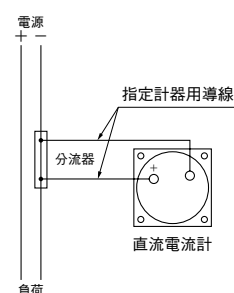
分流器外付の場合
